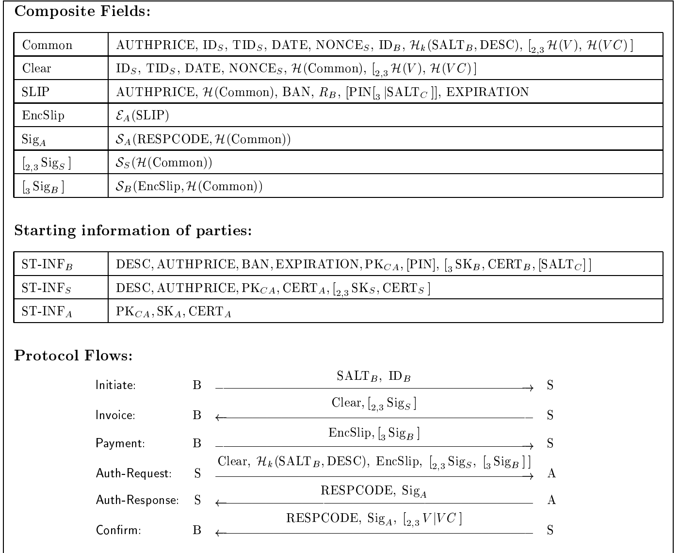
Fig. 5. iKP Protocols
